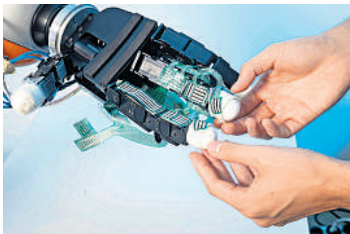
Les doigts de ce robot utilisé à l'EPFL sont couverts de capteurs tactiles, qui lui permettent de découvrir la forme des objets.
